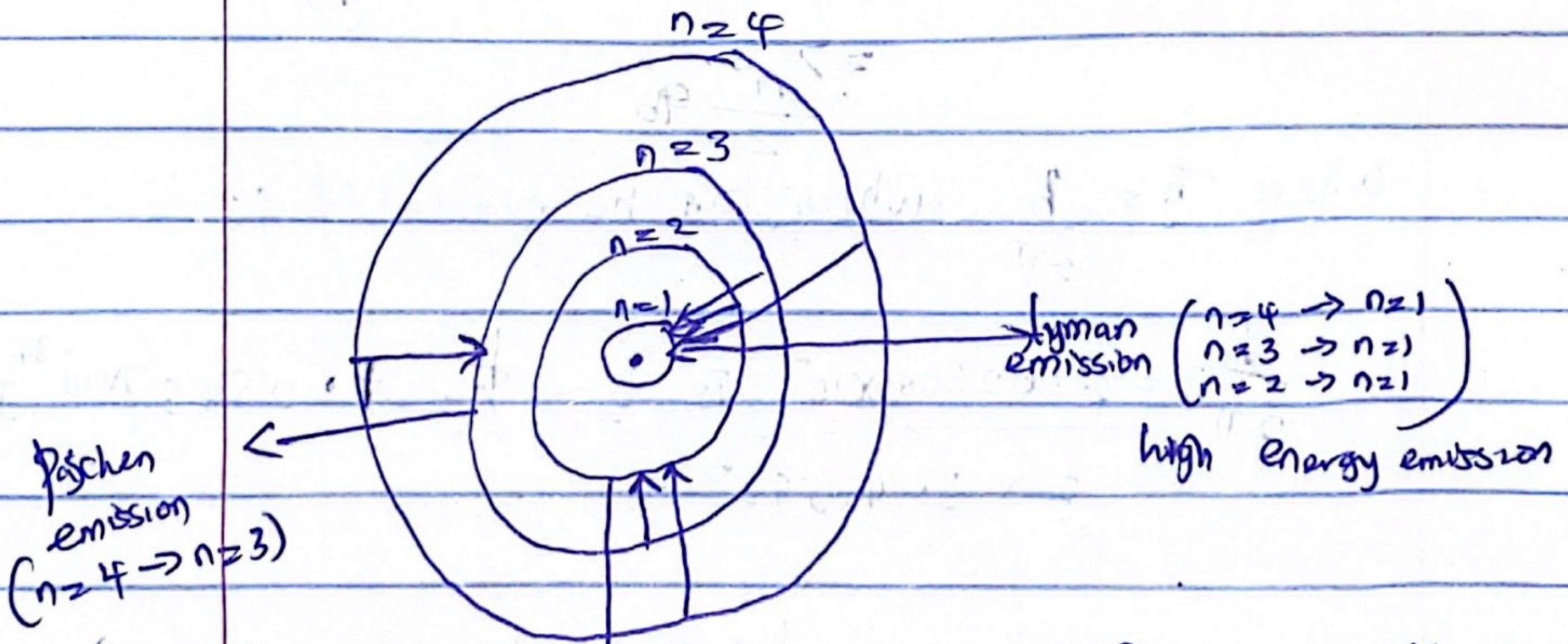
Fig A: Bohr Atomic model
